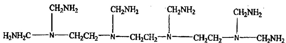
DTPA
