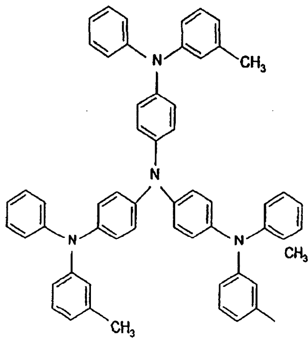
mTADATA
