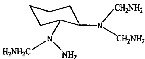
DETA
